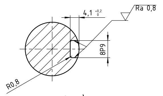
Presjek B-B (M 1:1)
