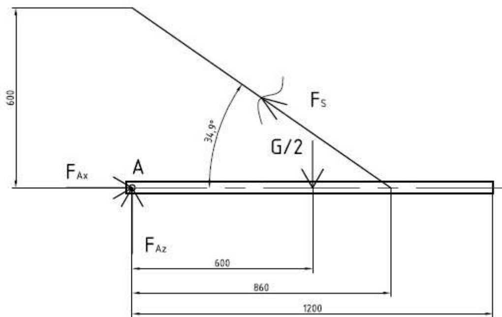
Slika 28. Shema opterećene platforme
