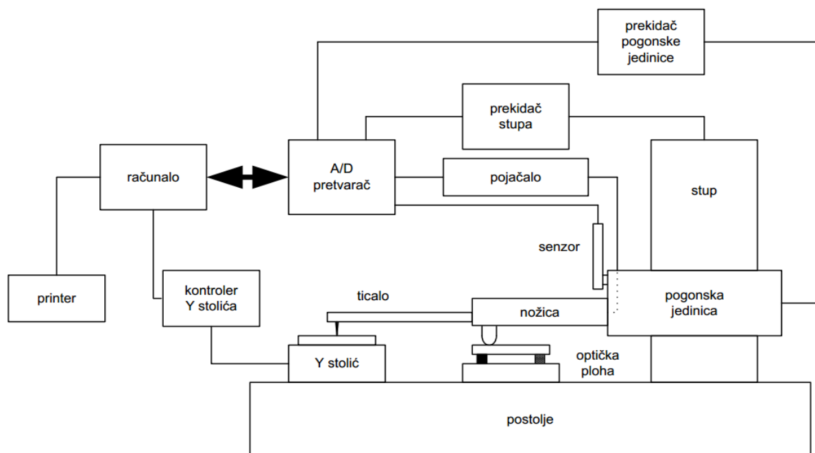
Slika 14. Konstrukcija ticala [17]
