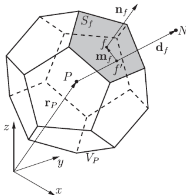
Slika 10. Kontrolni volumen
