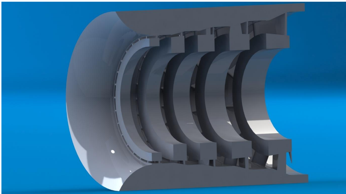
Slika 17. Stator mikroturbine
