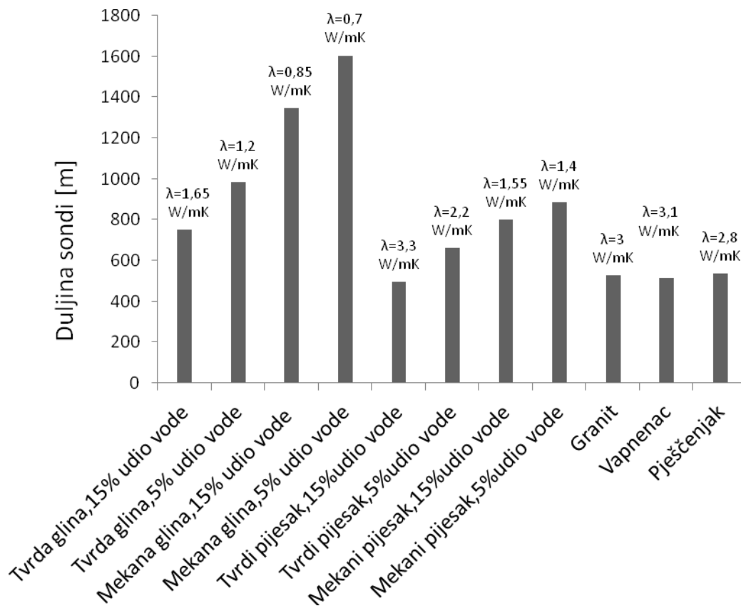
Slika 19. Utjecaj termofizikalnih karakteristika različitih tla na duljinu vertikalnih sonde
