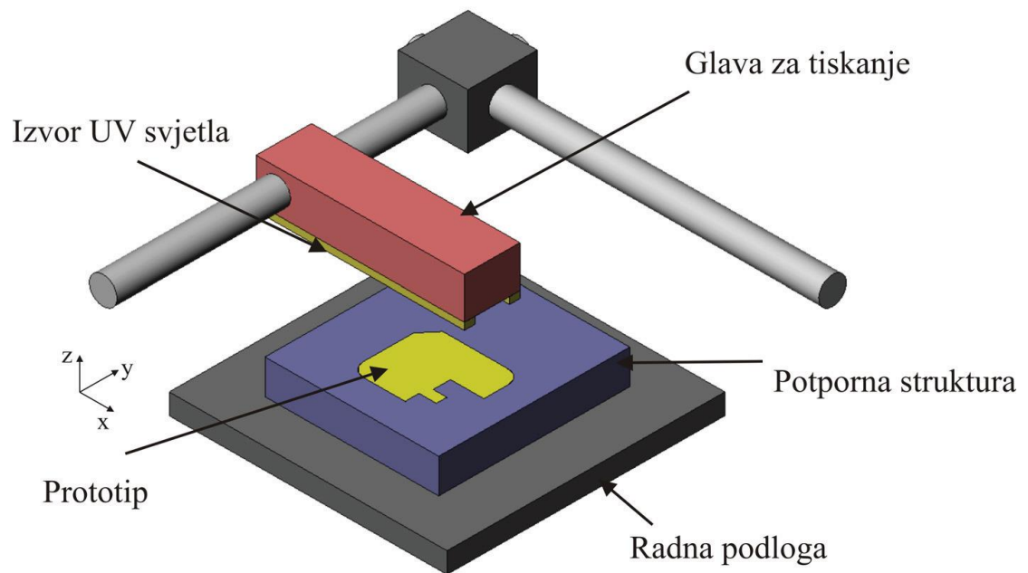
Slika 3.2 Polyjet postupak [1]
