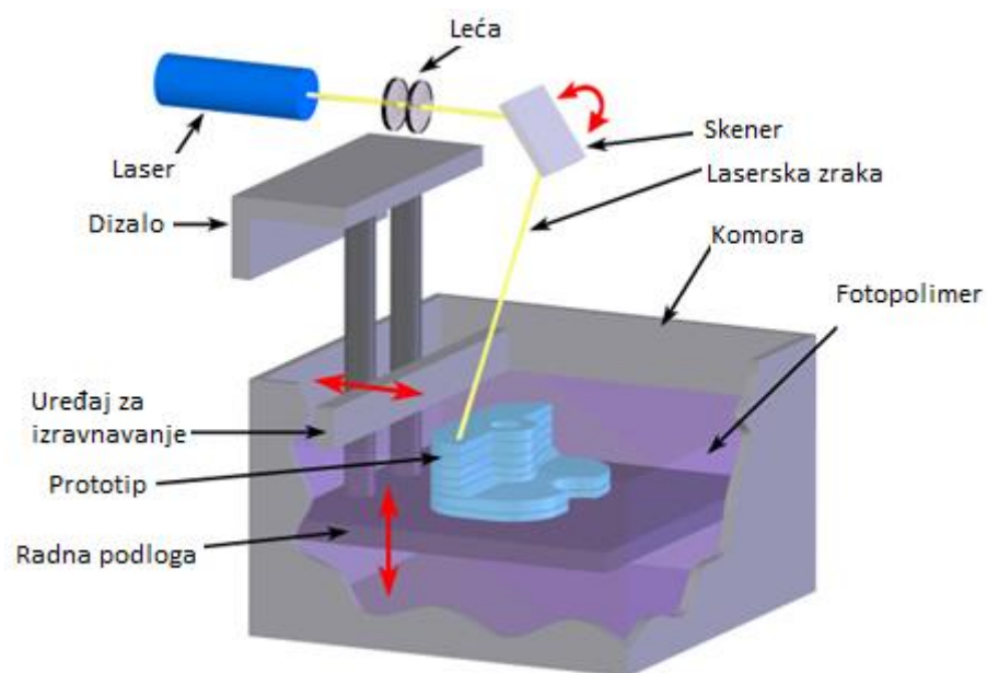
Slika 3.1 Postupak stereolitografije [4]
