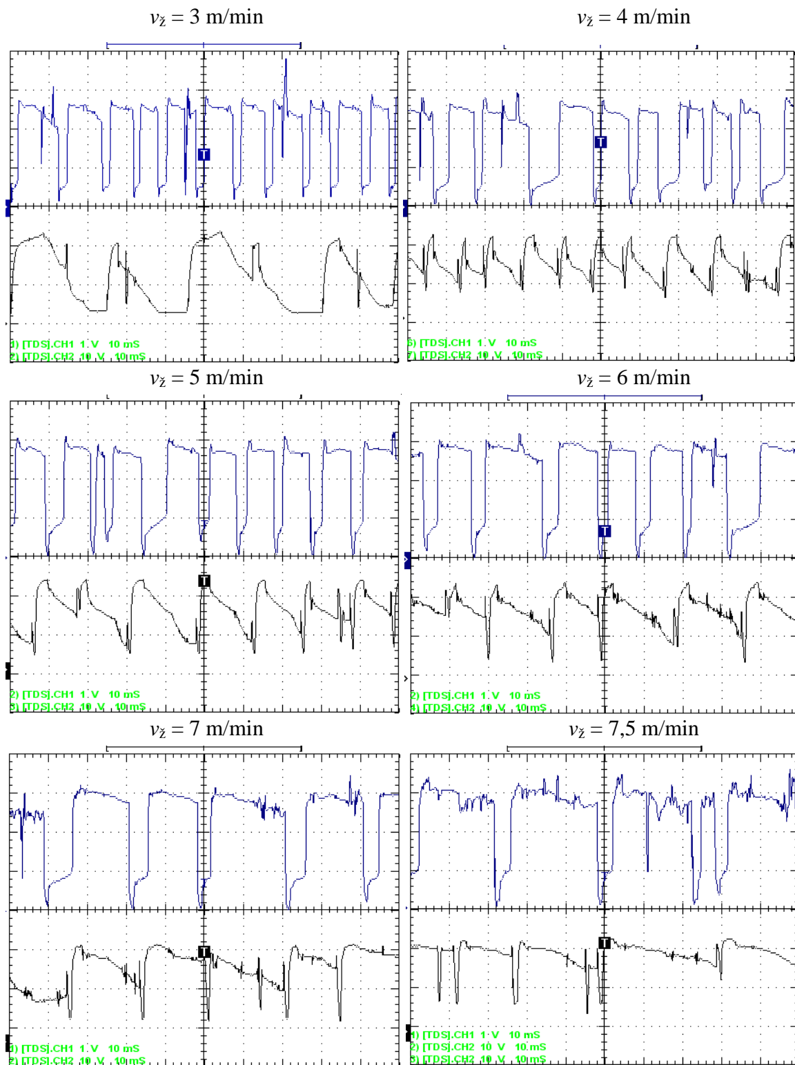
Slika 38. Oscilogrami dinamičkih karakteristika u_i = f(t) , pri klasičnom načinu prijenosa metala (100% CO 2 )
