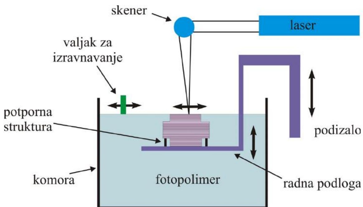
Slika 3.2. Postupak stereolitografije [9]
