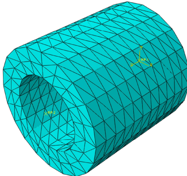
Slika 16. Diskretizirani model cijevi s tetraedarskim konačnim elementima
