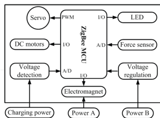
Slika 29. Hardver stanice za punjenje[8]
