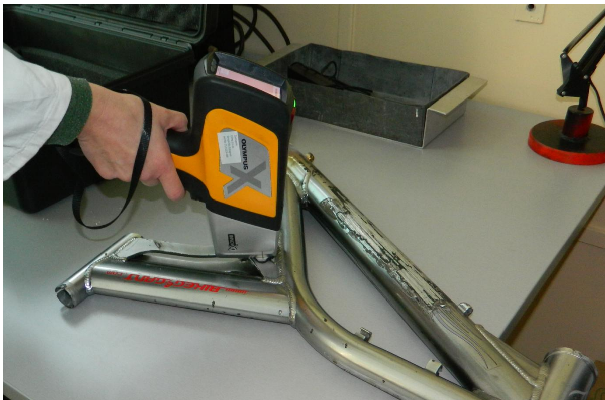
Slika 20. Određivanje masenog udjela kemijskih elemenata ručnim uređajem Olympus XRF
