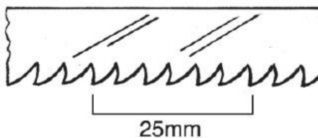
Slika 4. Broj zubi [5]
