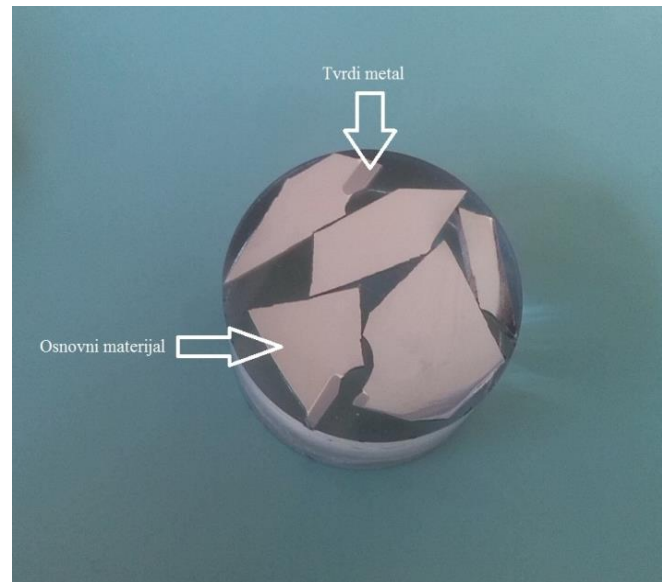
Slika 61. Pripremljeni uzorci
