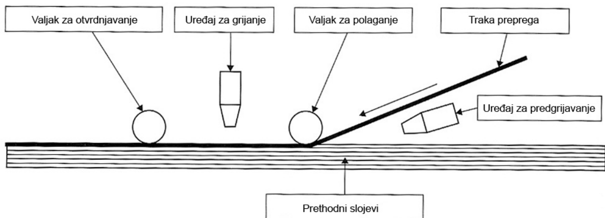
Slika 4.21. Drapiranje preprega [3]
