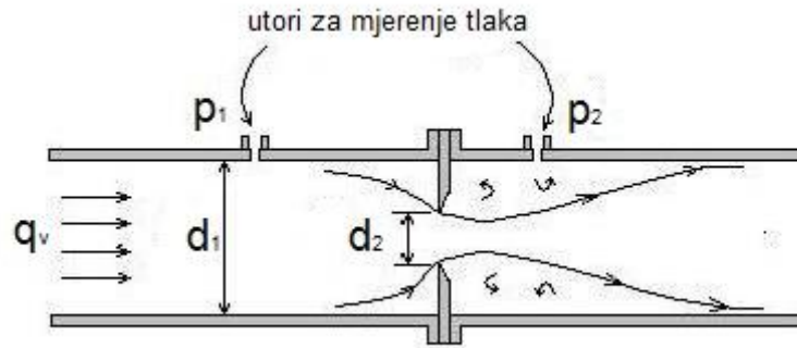
Slika 3. Mjerna prigušnica
