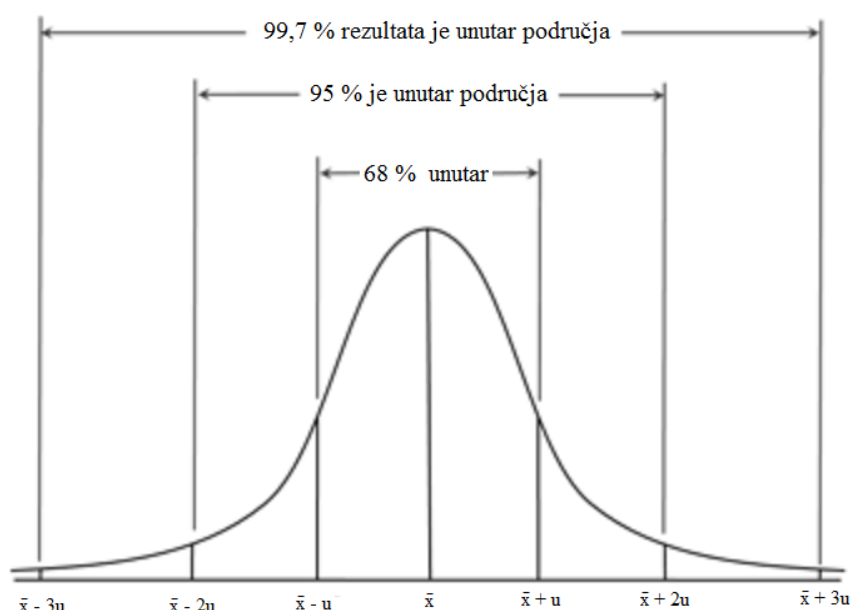
Slika 21. Gaussova razdioba
