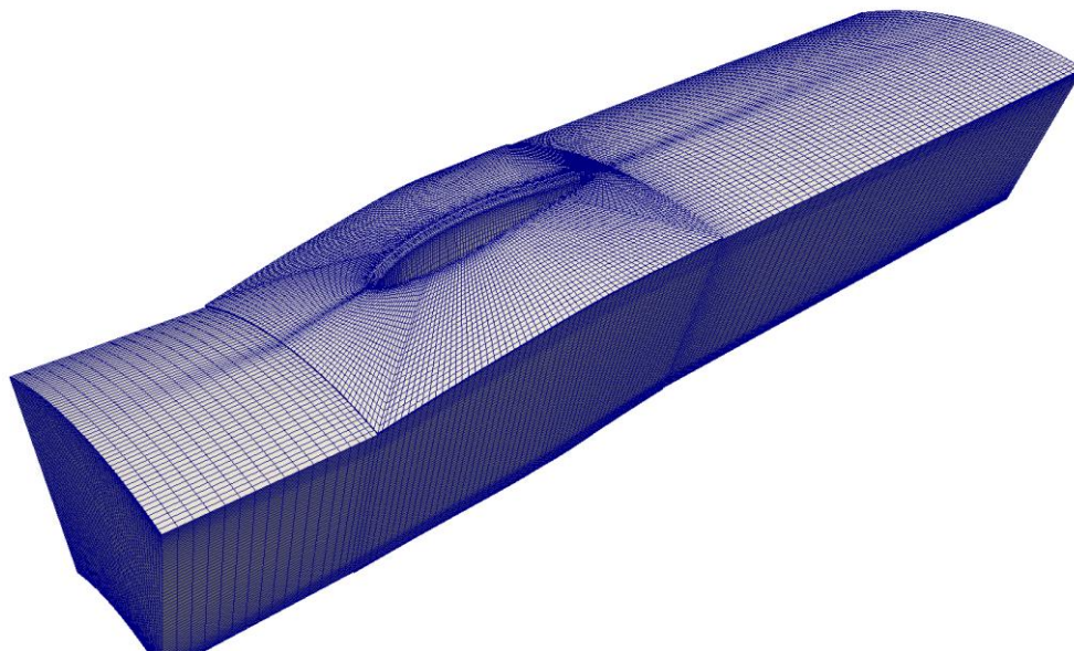
Slika 12 Mreža - fluid
