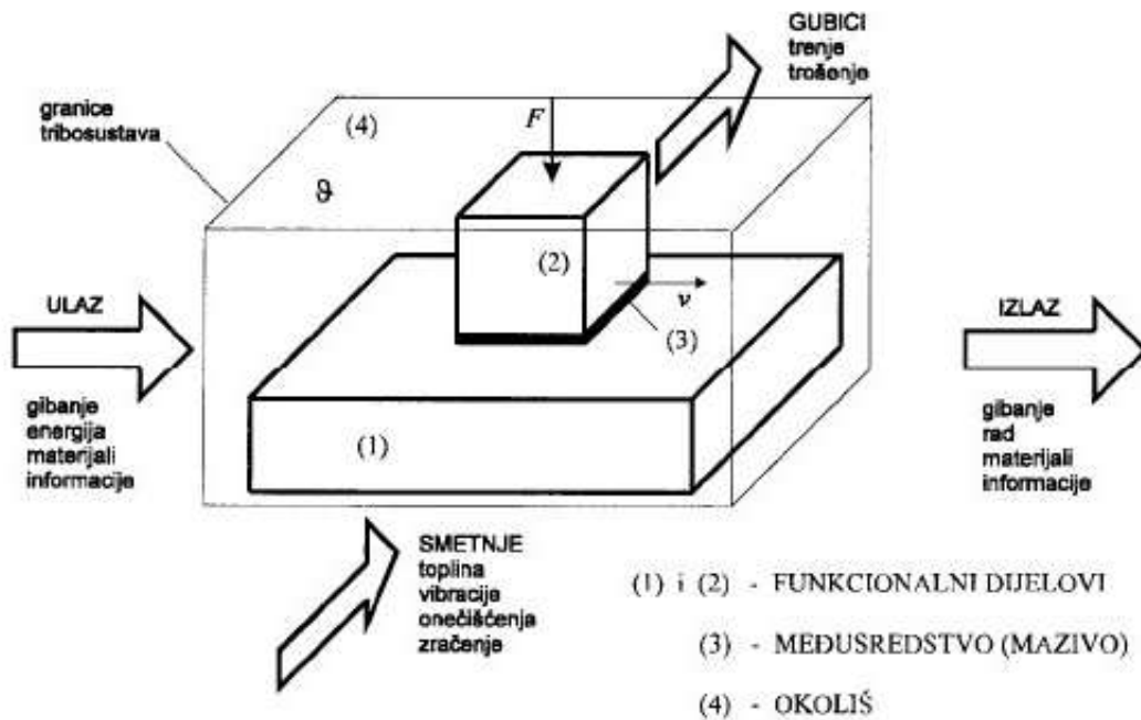
Slika 15. Elementi tribosustava [20]
