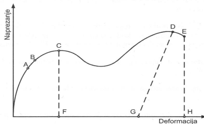
Slika 5.5. Opći dijagram napreznje-deformacija: A – granica proporcionalnosti, B – granica elastičnosti, C – granica tečenja, D – čvrstoća pri djelovanju maksimalnog opterećenja, E – nominalno napreznje pri djelovanju sile koj razdvaja dijelove ispitka, F – deformacija pri granici tečenja, G – trajna deformacija po rasterećenju, H – ukupna deformacija [2]
