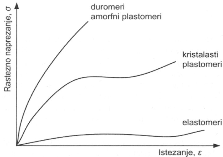
Slika 5.2. Karakteristični dijagrami rastezno naprežanje-istežanje osnovnih skupina polimernih materijala [2]
