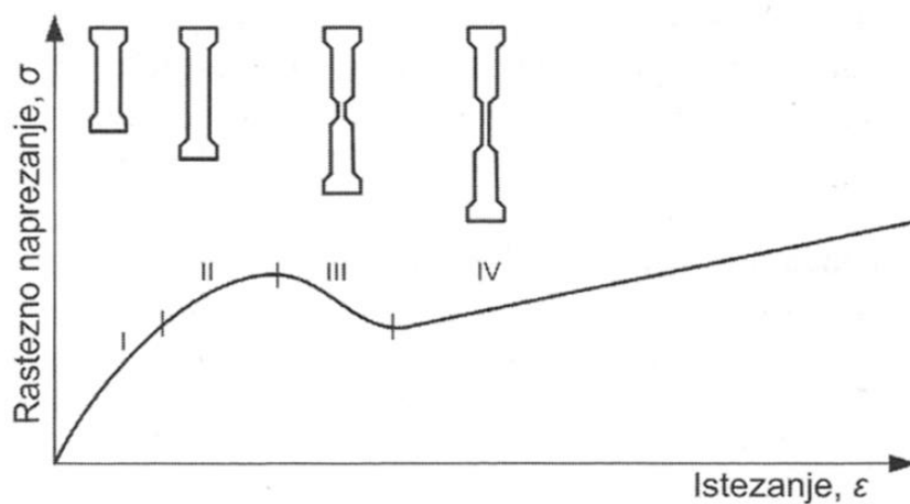
Slika 5.3. Raščlanjeni dijagram rastezno naprežanje-istežanje kristalastih plastomera [2]
