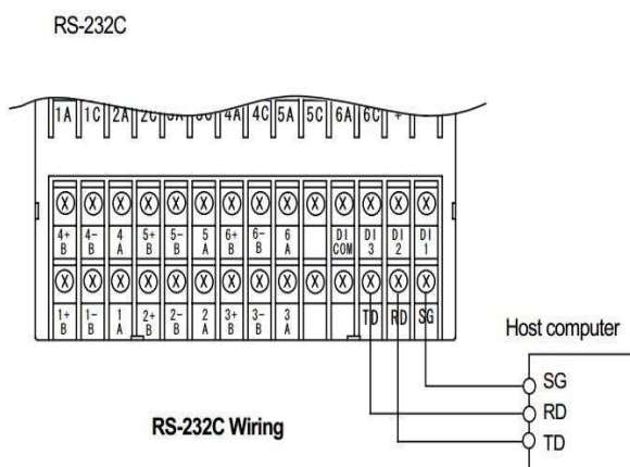
Slika 36. Shema spajanja računala s registratorom temperature
