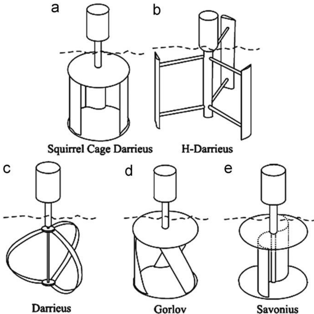
Slika 4. Vertikalnealne turbine [2]
