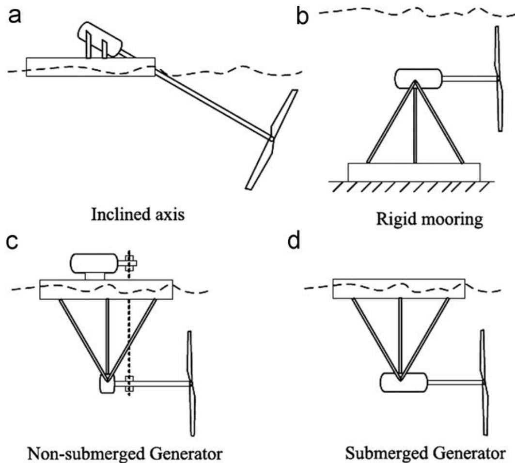
Slika 1. Horizontalne hidroturbine [2]
