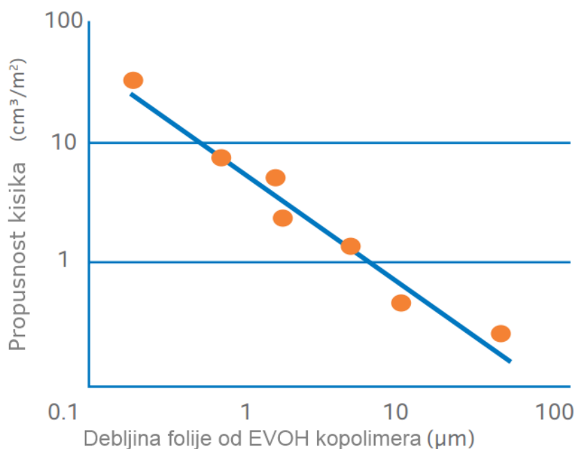
Slika 4. Propusnost kisika u odnosu na debljinu folije EVOH kopolimera pri temperaturi od 35 °C i 0% relativne vlažnosti zraka u trajanju od 24h pri atmosferskom tlaku [1]
