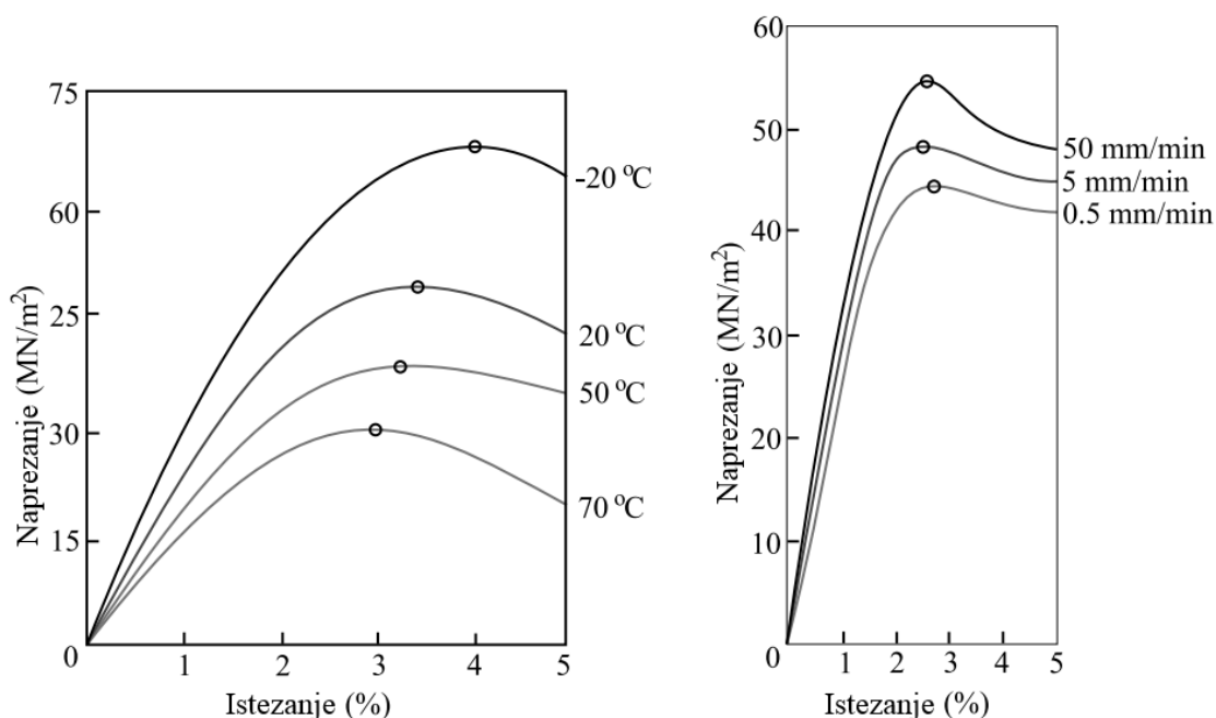
Slika 25. Tipični dijagrami naprezanje-istezanje za različite brzine istezanja i za različite temperature kod polimera [35]
