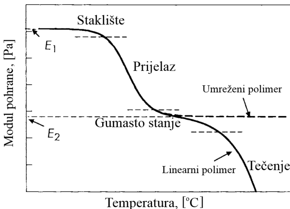
Slika 32. Shematski dijagram modula elastičnosti u ovisnosti o temperaturi koji pokazuje različita područja viskoelastičnog ponašanja [34]
