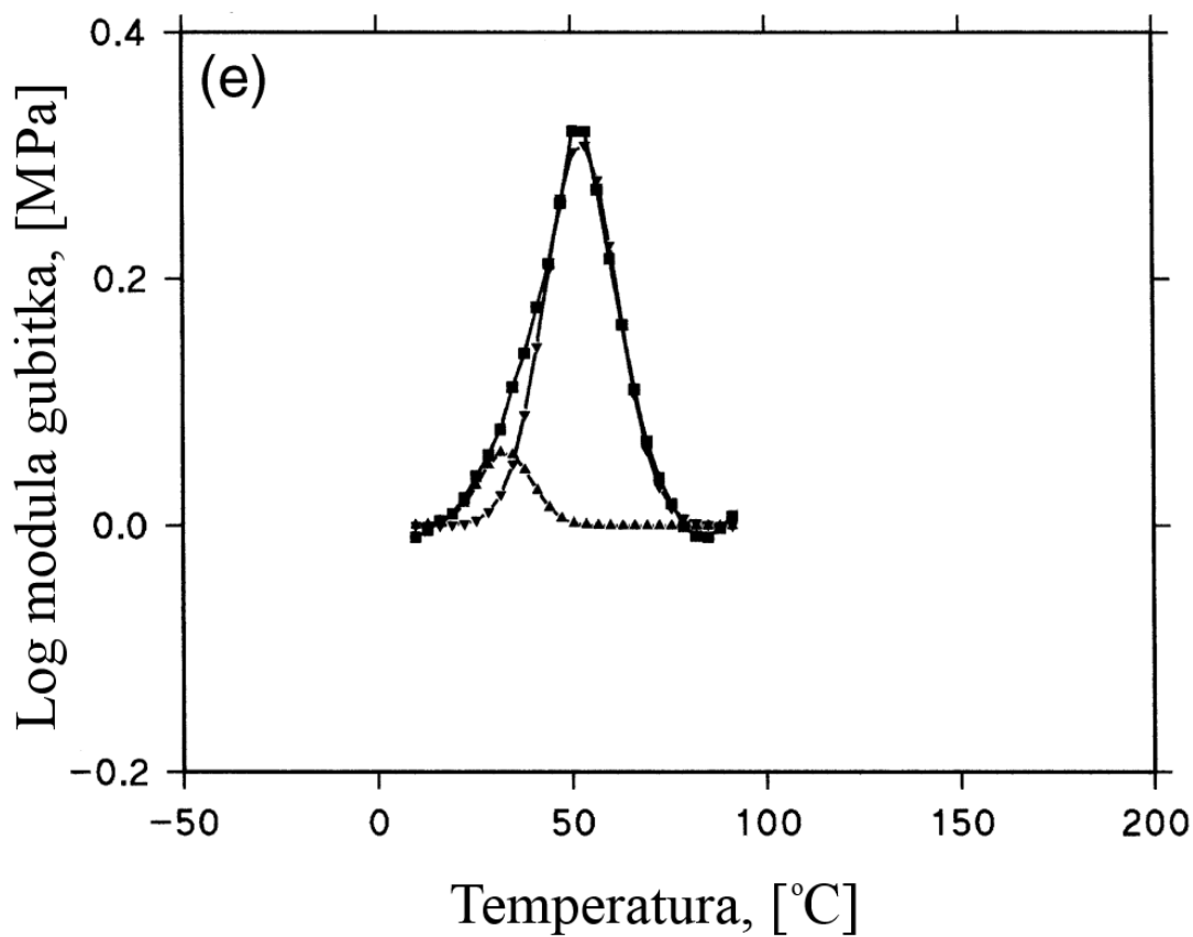
Slika 35. Modul gubitka E'' folije od EVOH kopolimera koji sadrži oko 29 mol% etilena pri rasteznom naprezanju frekvencije 1 Hz, bez prednaprezanja. Zadana amplituda istezanja je 16 \mu\text{m} . [43]
