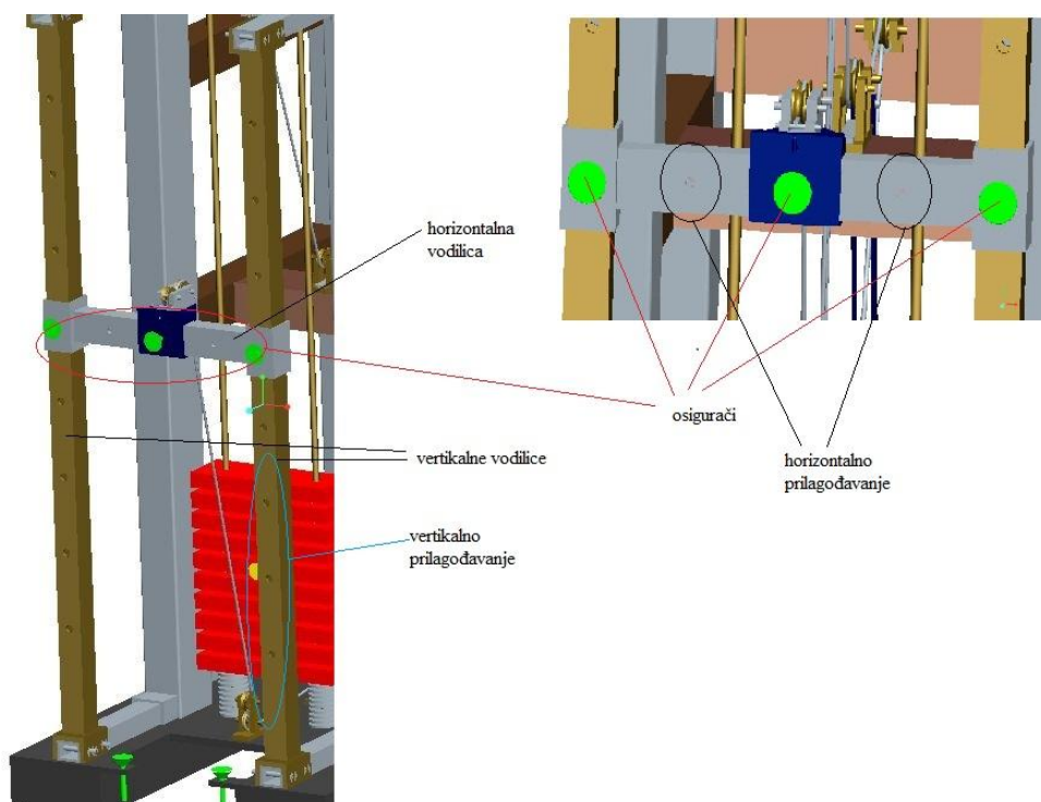
Slika 50 Podešavanje početnog položaja naprave
