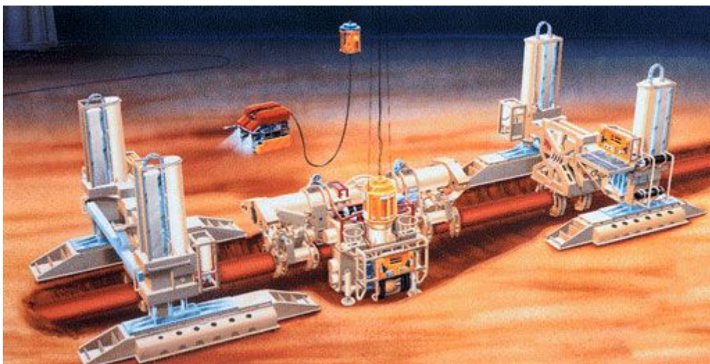
Slika 2.3.2 Podvodni habitat; sustav za popravak cjevovoda uključuje takozvane habitat module koji omogućuju ronionicima rad u suhom okruženju na dnu mora [37]
