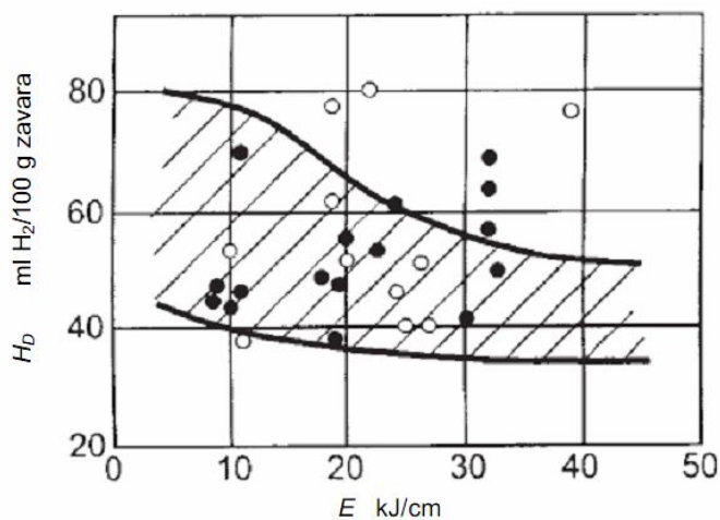
Slika 2.4.3 Utjecaj unosa topline na količinu difundiranog vodika pri mokrom
