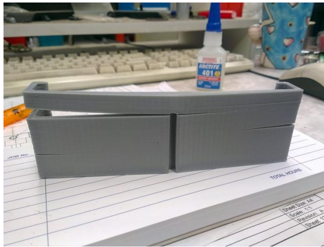
Slika 3.32 Raslojavanje modela zbog preniske temperature [50]
