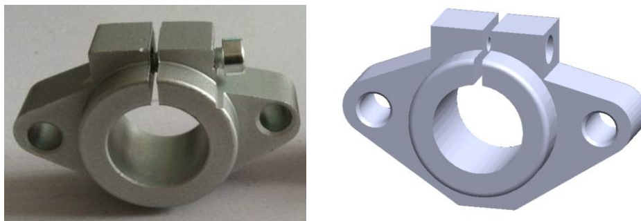
Slika 5.9 Držač osovine (SHF 16) [78]
