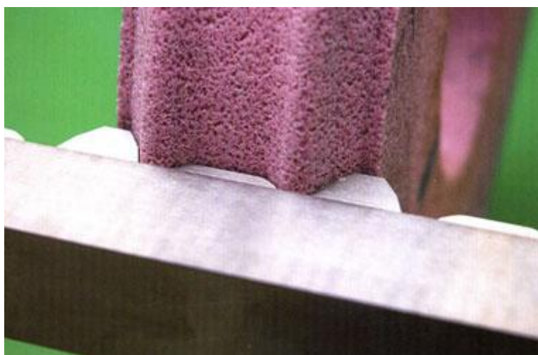
Slika 22. Primjer dubokog brušenja [14]
