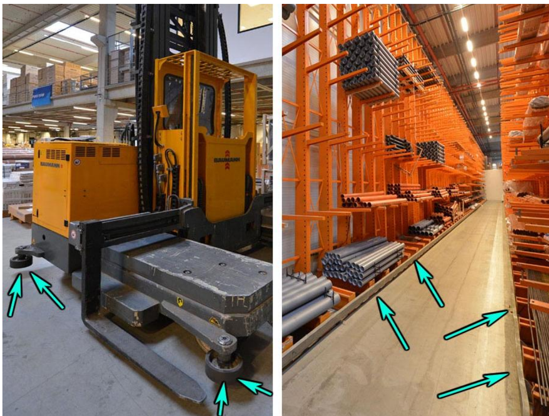
Slika 56. Vodilice četverostranog viličara u prolazu s konzolnim regalima u skladištu poduzeća Feroterm
