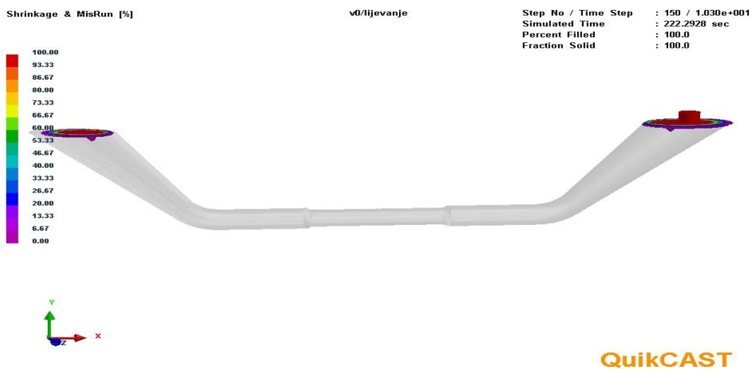
Slika 27. Poroznost odljevka
