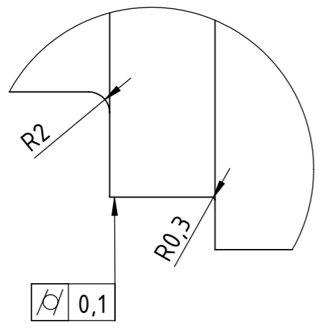
DETALJ A 2 : 1
