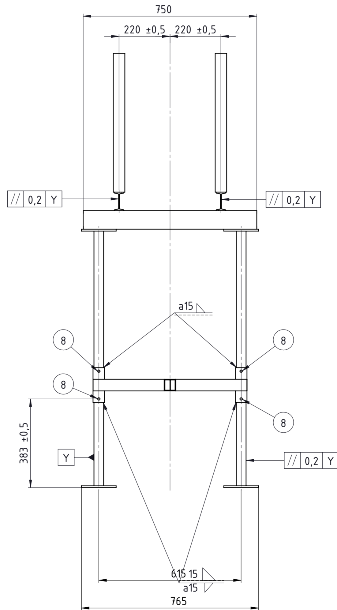
PRESJEK A-A 1 : 10
