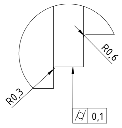
DETALJ B 2 : 1
