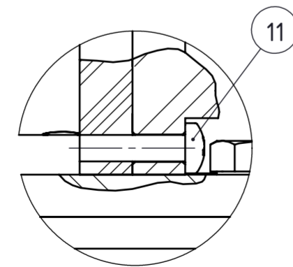
DETALJ A 1 : 1
