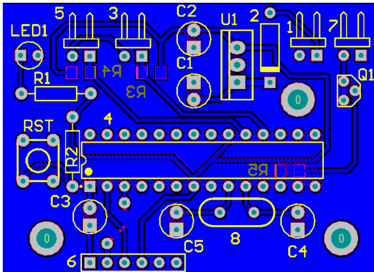
Slika 39: PCB pločice
