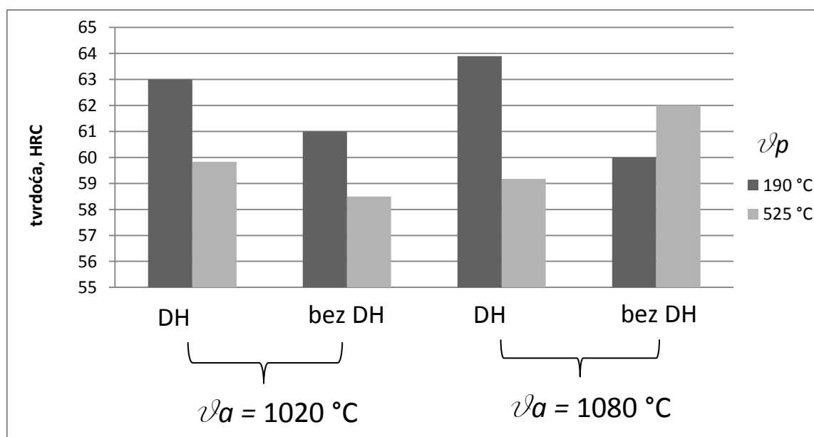
Slika 23. Tvrdoće uzoraka
