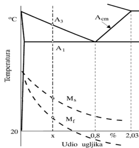
Slika 14. Uptonov dijagram
