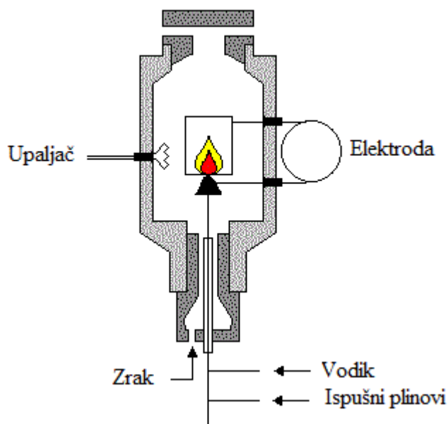
Slika 6.6 FID sustav
