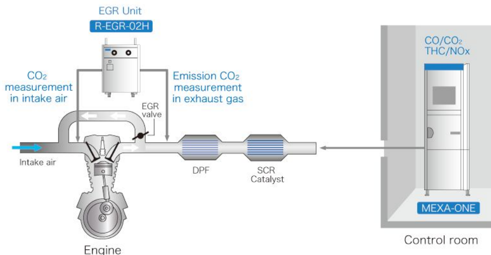
Slika 6.4 EGR mjerenje [30]
