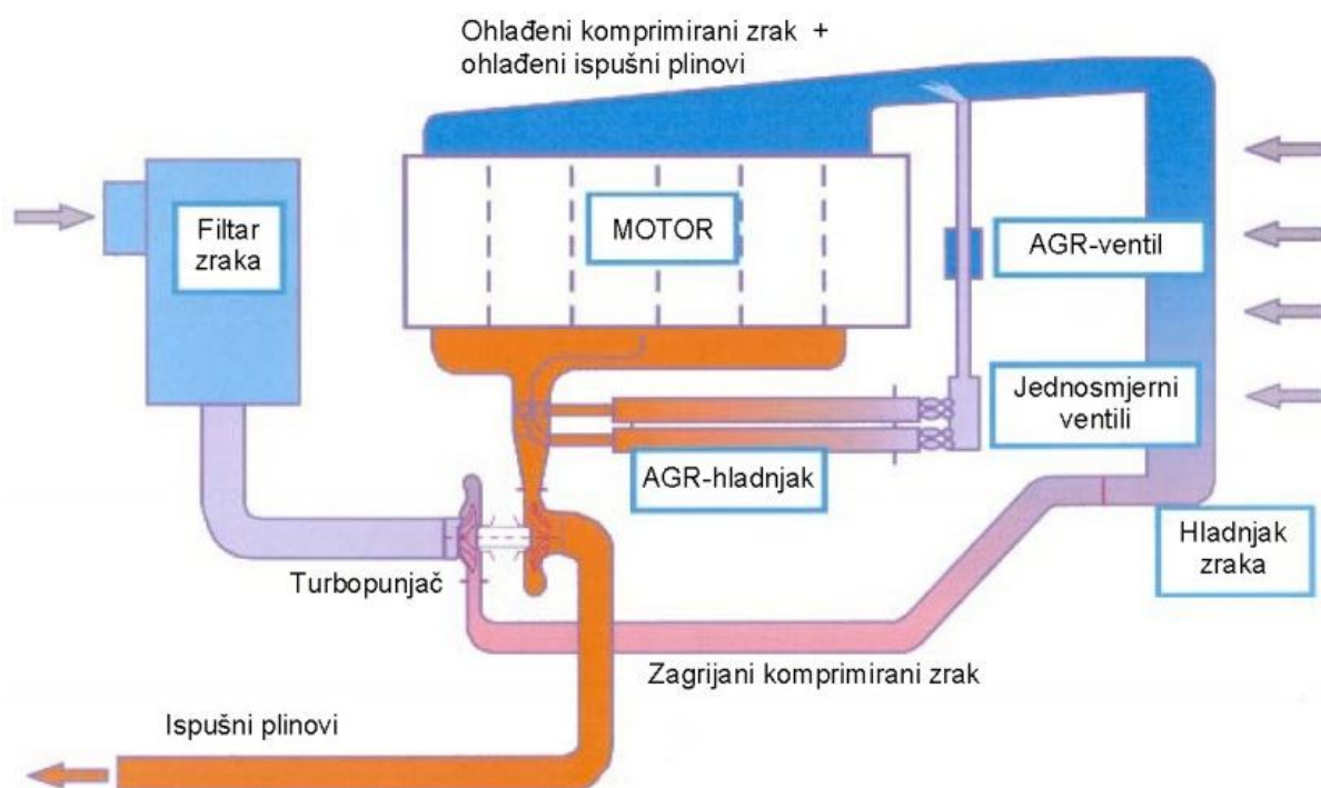
Slika 4.7 EGR sustav[3]
