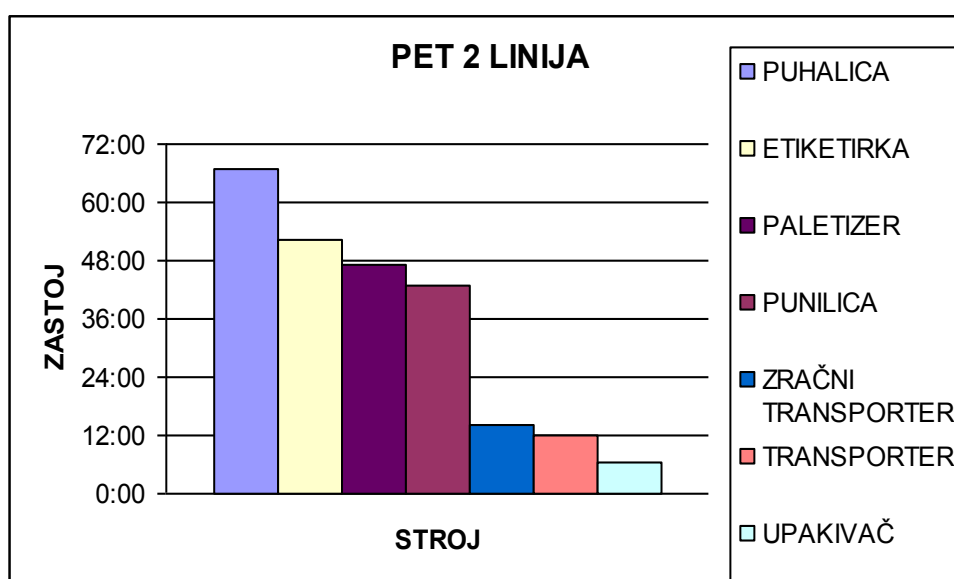
Slika 8.9. Zastoji PET 2 linije izražen u satima
