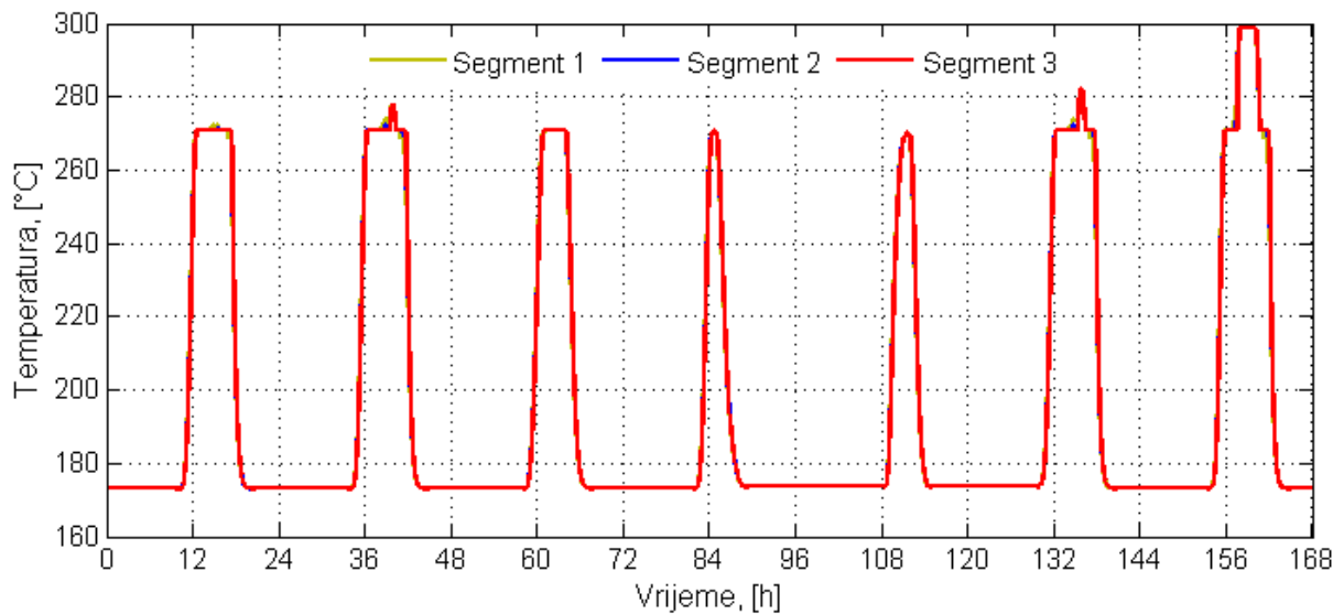
Slika 49. Temperature PCM-a u četvrtom odsječku
