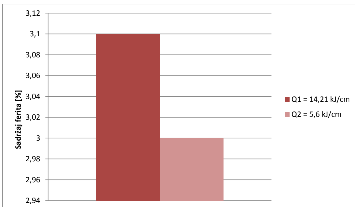
Slika 24. Sadržaj ferita pojedinog unosa topline
