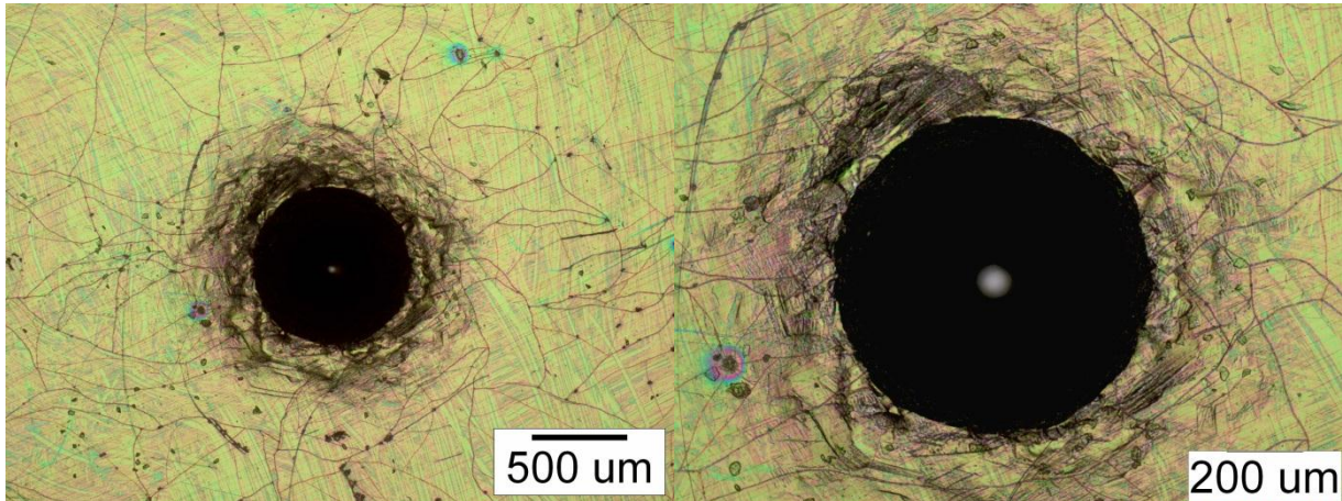
Slika 29 - Površina uzorka \text{TiO}_2\text{-ZrO}_2 2 B (povećanje lijevo 50x i desno 100x)
