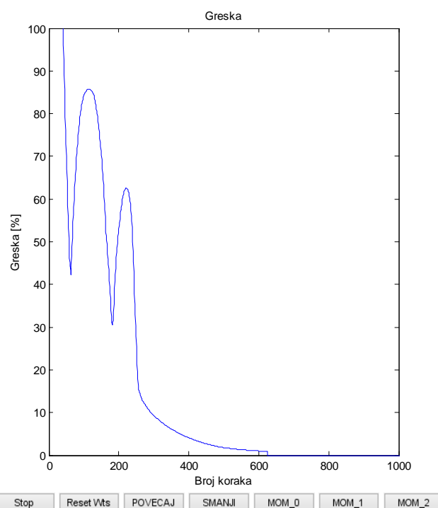
Slika 16. Rezultat učenja nelinearne funkcije f(x) = \sin(3 \cdot x) / x
