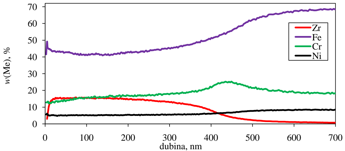
Slika 37. Kvantitativna dubinska profilna analiza (GDS-QDP) sol-gel \text{ZrO}_2 filmova na nehrđajućem čeliku, ovisnost atomskih udjela pojedinih elemenata (%) o dubini (nm) kod uzorka 3C-GORE ( \vartheta_k = 600 °C, \alpha = 30^\circ , 500 udaraca)
