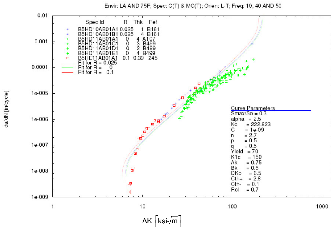
Slika 36. Ovisnost brzine širenja pukotine o \Delta K za čelik A533-B [4]
