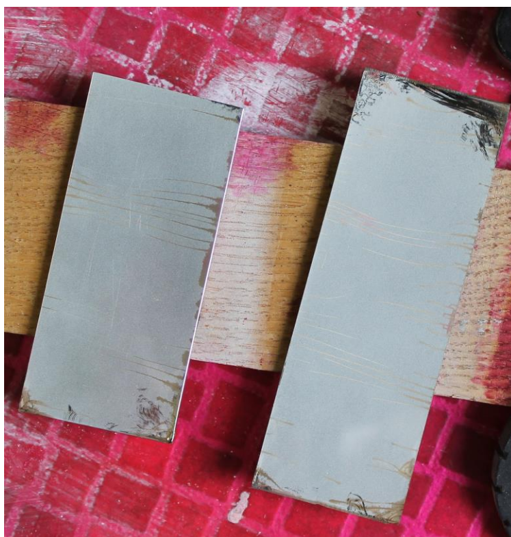
Slika 24. Indikacije na površinama etalona (gornja slika: T_{\text{pen}}=15 min, T_{\text{raz}}=20 min, E=300 lx, \vartheta=80^{\circ}\text{C} donja slika : T_{\text{pen}}=15 min, T_{\text{raz}}=20 min, E=800 lx, \vartheta=80^{\circ}\text{C} )
