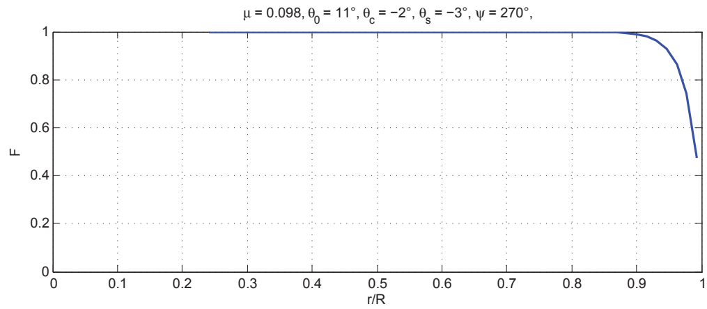
Slika 26 – Koeficijent gubitaka na vrhu kraka po rasponu kraka
