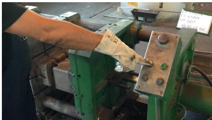
Slika 30. Probni rad nove kokile (provjeravanje centriranosti)
