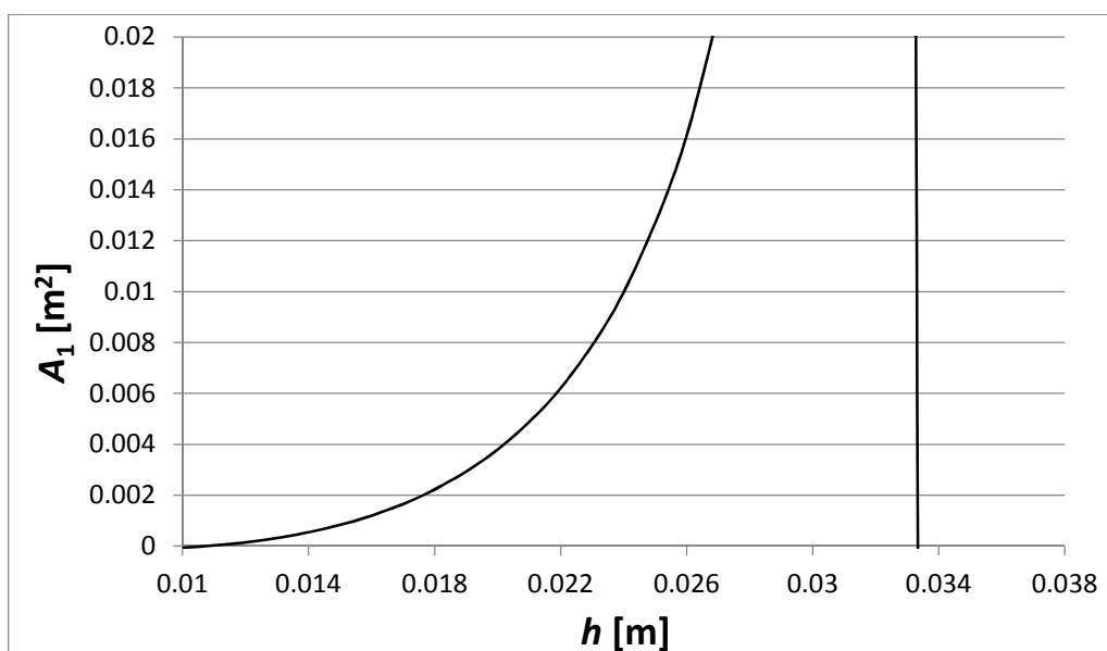
Slika 18. Grafički prikaz ovisnosti funkcije ograničenja meridijalnog napreznja o debljini oplata
