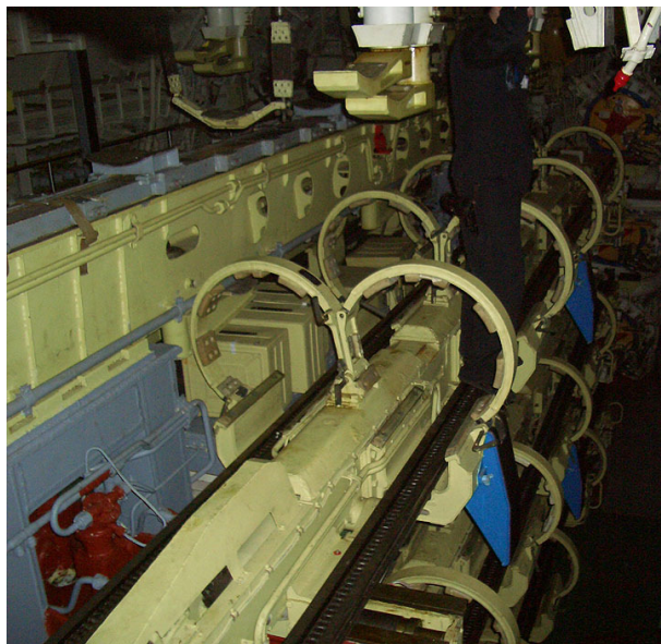
Slika 40. Sustav za automatsko punjenje torpeda ugrađen na Typhoon klasi [37]
