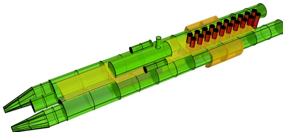
Slika 83. Prikaz svih prostora koji sudjeluju u uzgonu nakon balastiranja za oštećenje 6
