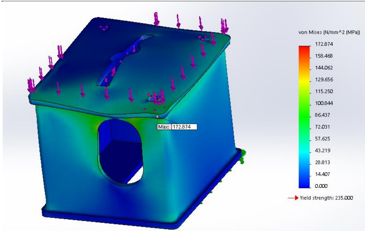
Slika 43. Maksimalna naprezanja
