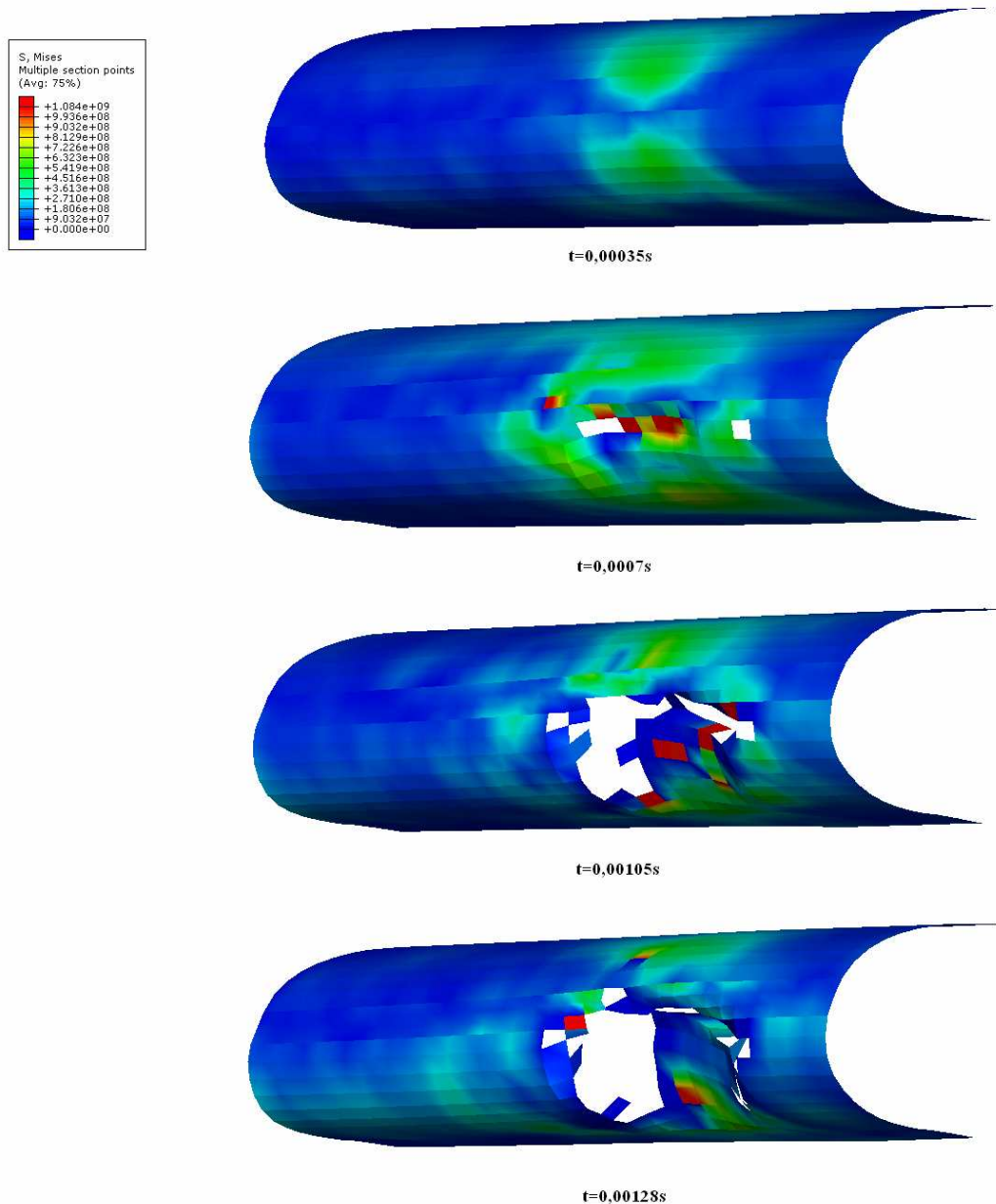
Slika 4.10. Raspodjela ekvivalentnog Von Mises naprezanja na vanjskoj oplati sandwich konstrukcije, mjesto udara 1 pod 40^\circ
