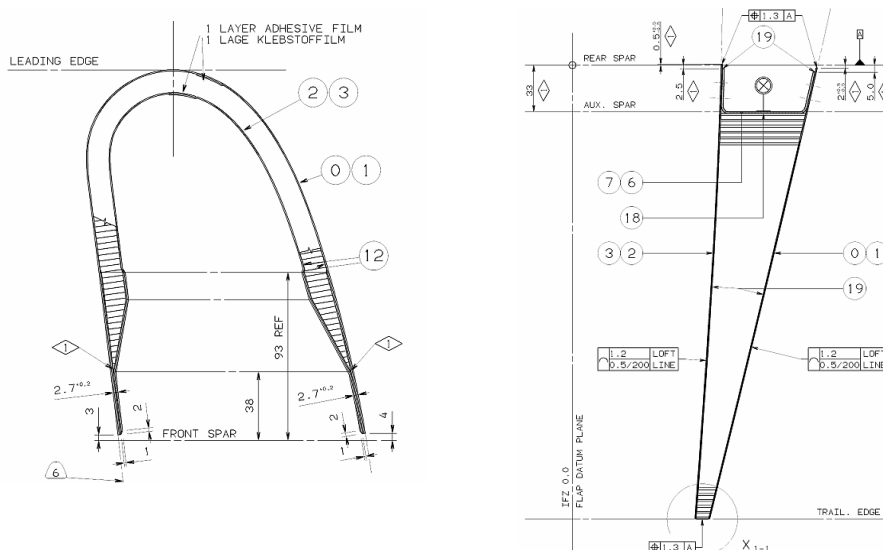
Slika 2.9 Prikaz sandwich konstrukcije napadnog (lijevo) i izlaznog (desno) ruba [2]
