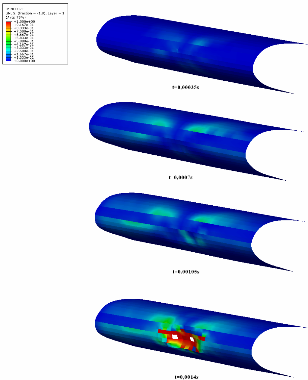
Slika 4.23 Vrijednost indeksa Hashinog kriterija popuštanja u prvom sloju unutarnje oplata sandwich konstrukcije za slučaj udara u mjesto 1 pod kutem od 60°
