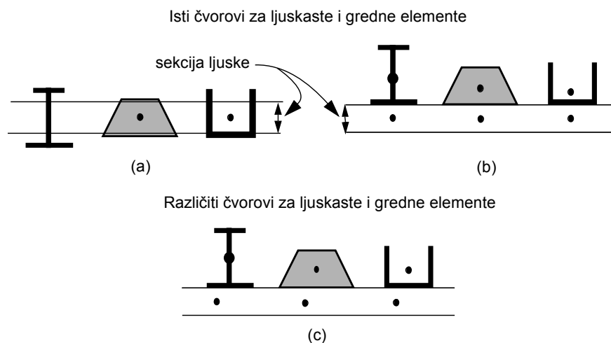
Slika 2.16 (a) gredni elementi u ravnini s luskastim, dijele čvorove; (b) gredni elementi odmaknuti na površinu ljuski, čvorovi se vertikalno poklapaju; (c) gredni elementi odmaknuti, čvorovi se ne poklapaju [6]
