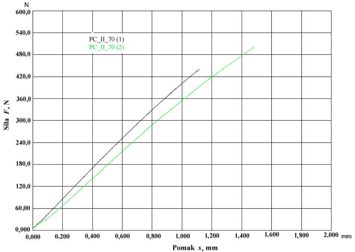
Slika 6.14. Dijagram sila – pomak za ispitno tijelo PC_II_70
