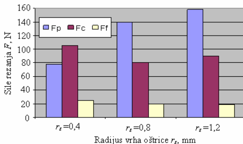
Slika 28. Ovisnost sile rezanja o radijusu vrha reznog alata [16]
