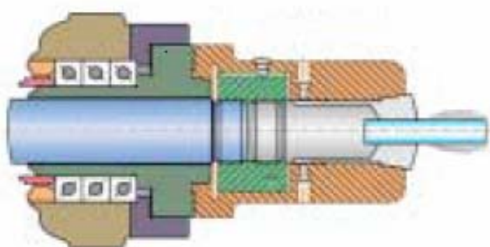
Slika 23.b) Glavno vreteno na uobičajenim tokarilicama [16]
