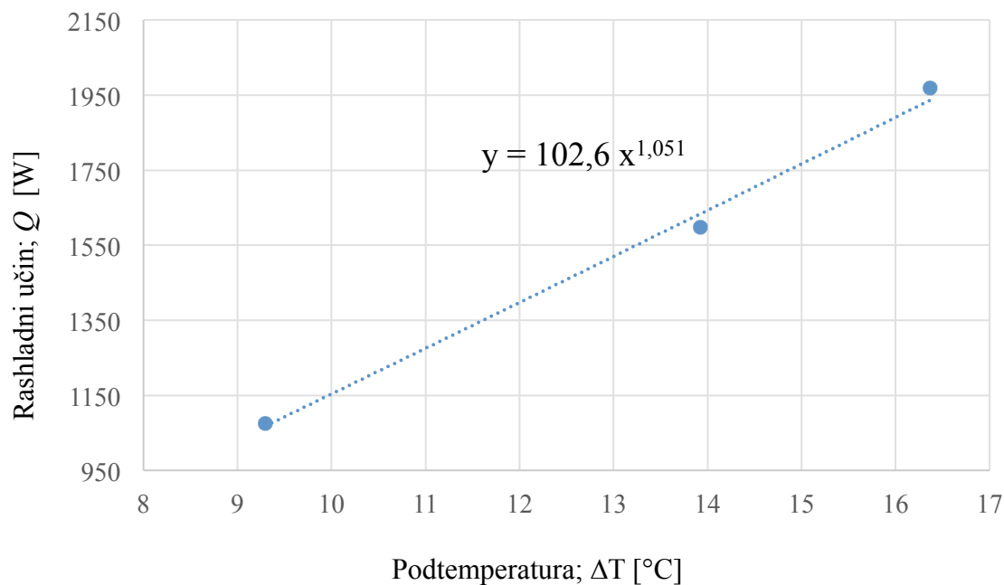
Slika 82. Toplinska karakteristika pri brzini ventilatora 3
