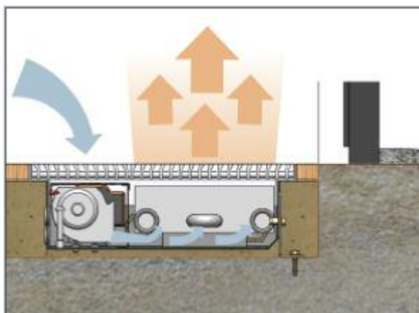
Slika 9. Podni ventilokonvektor
