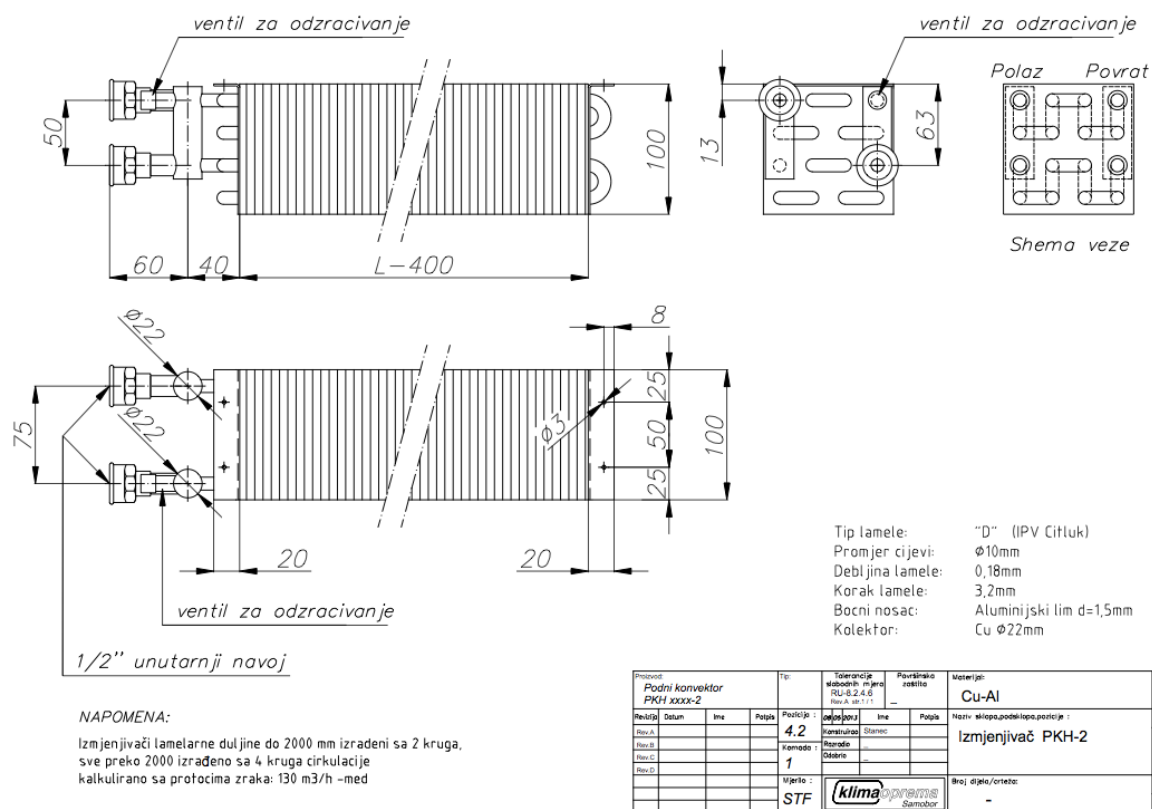
Slika 23. Shema izmjenjivača ispitivanog ventilokonvektora
