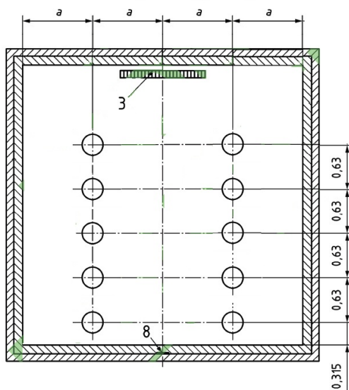
Slika 20. Ispitna prostorija s postavljenim konvektorom i grijačima
