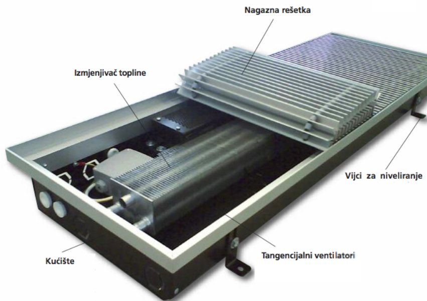
Slika 7. Konstrukcijski elementi podnog konvektora
