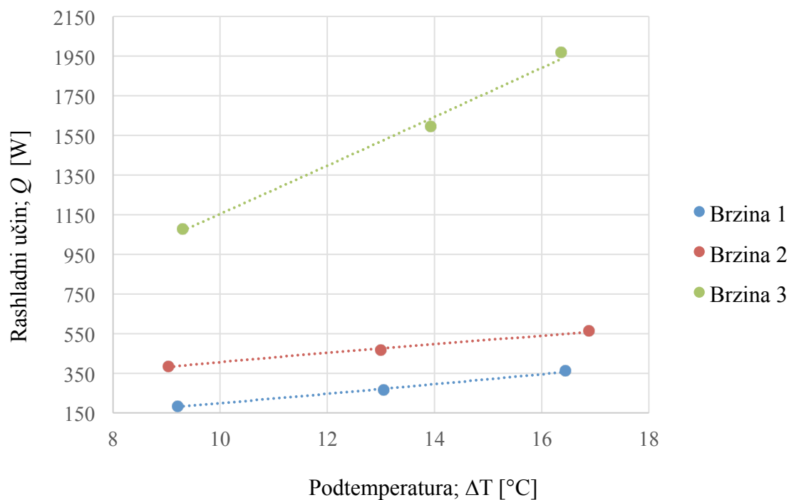
Slika 83. Usporedba toplinskog učina prema brzini ventilatora
