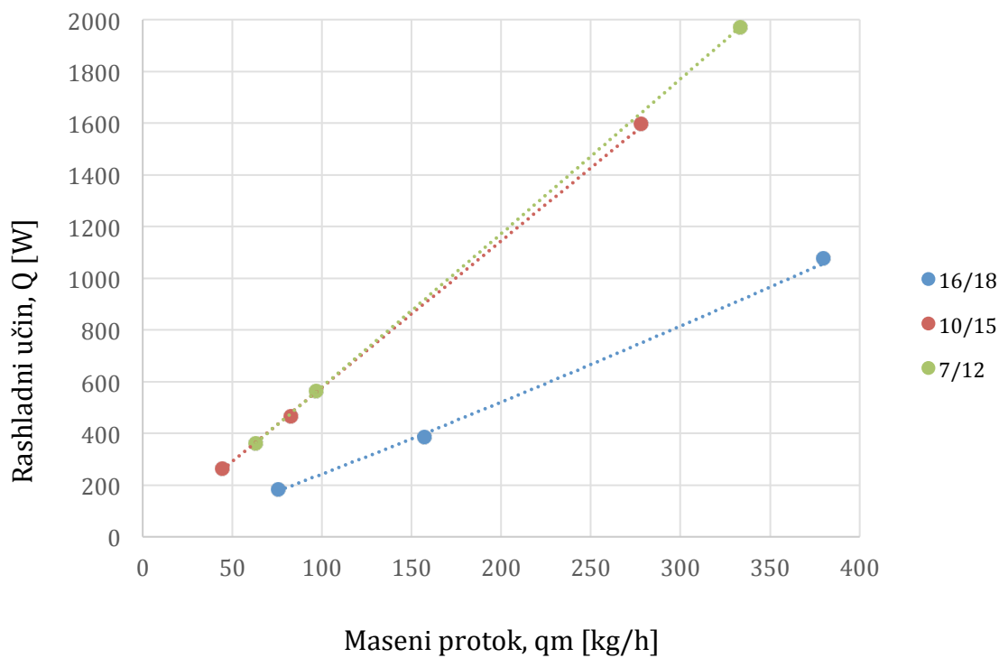
Slika 84. Usporedba toplinskog učina prema temperaturnom režimu
